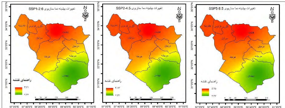
شکل ۳- تغییرات دمای بیشینه در طی دوره (۲۱۰۰ - ۲۰۲۰) تحت سناریوهای SSP1-2.6، SSP2-4.5 و SSP5-8.5 به درجه سلسیوس
