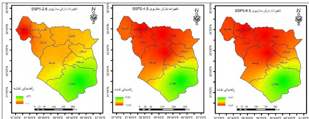
شکل ۲- تغییرات بارش طی دوره (۲۱۰۰ - ۲۰۲۰) تحت سناریوهای SSP1-2.6، SSP2-4.5 و SSP5-8.5 به درصد
